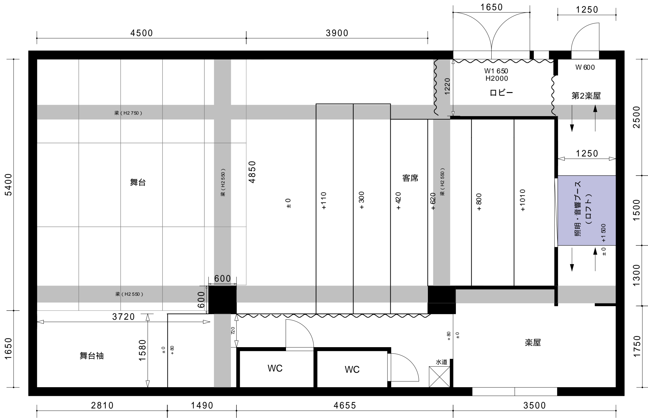
劇場平面図
